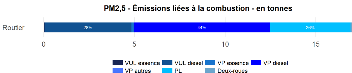
Figure 12 | Jalle Eau Bourde – PM2,5, émissions du secteur des transports, en tonnes
