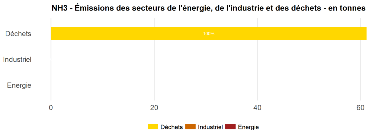
Figure 29 | Jalle Eau Bourde – NH 3 , émissions des secteurs de l'énergie, de l'industrie et des déchets, en tonnes
