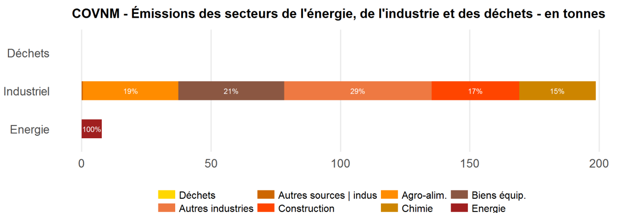
Figure 20 | Jalle Eau Bourde – COVNM, émissions des secteurs de l'énergie, de l'industrie et des déchets, en tonnes
