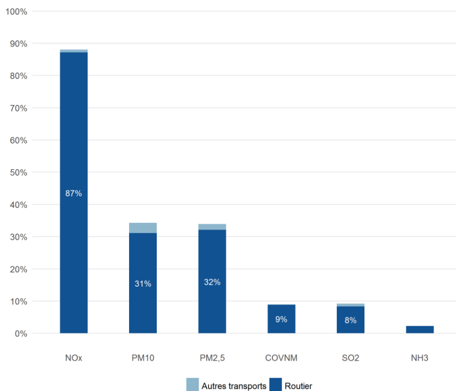
Figure 30 | Jalle Eau Bourde, Contribution des secteurs d'activités aux émissions polluantes
