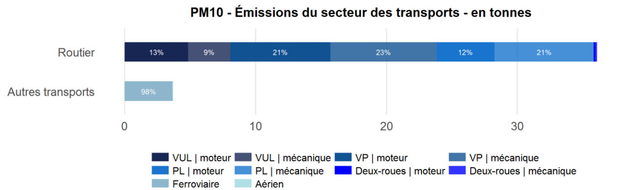
Figure 10 | Jalle Eau Bourde – PM10, émissions du secteur des transports, en tonnes
