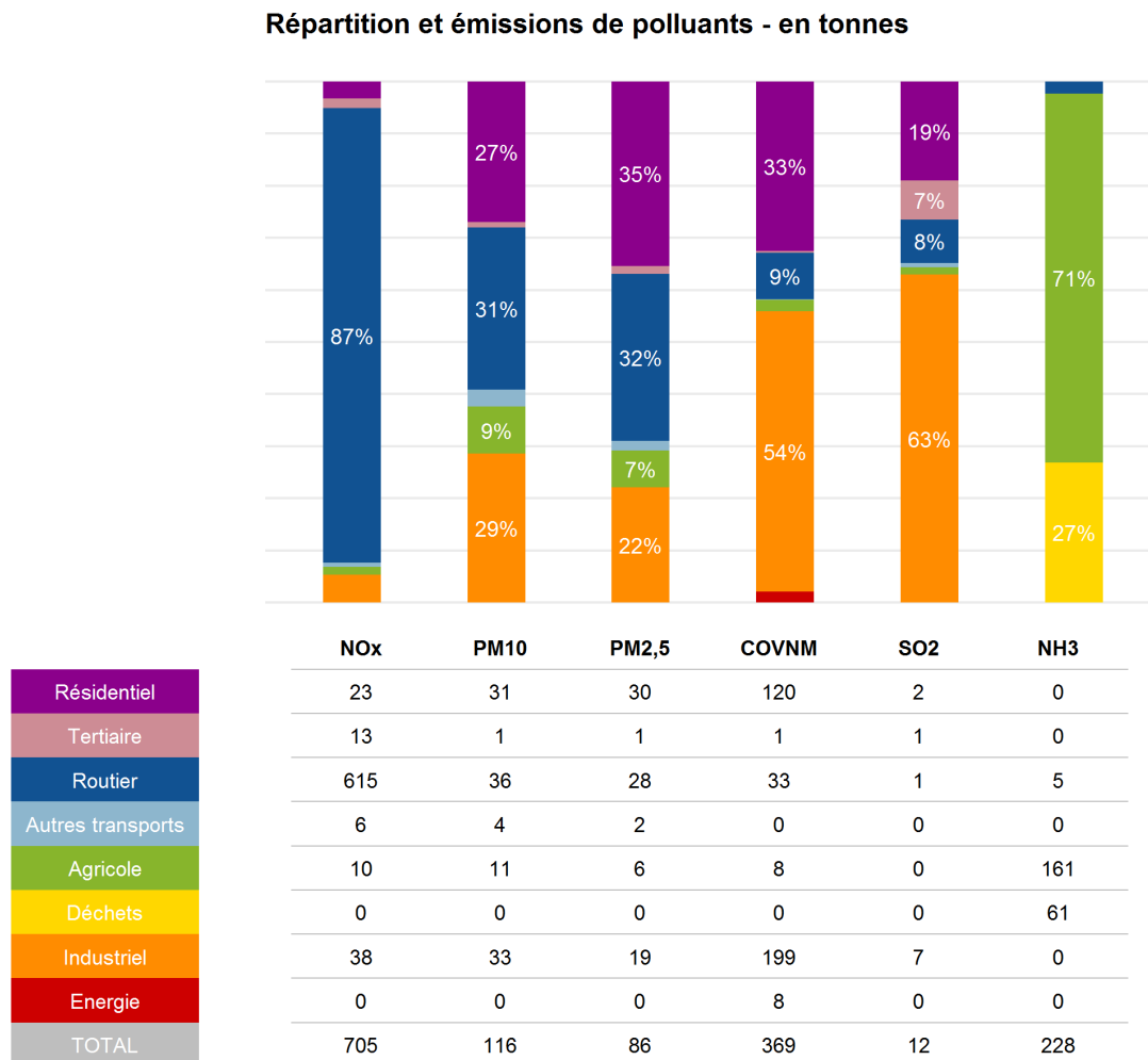
Figure 3 | Jalle Eau Bourde - Répartition et émissions de polluants par secteur, en tonnes
